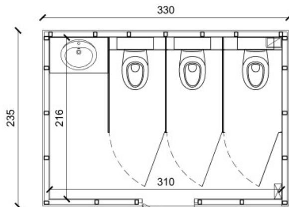
C « Femmes » (3 WC, 1 lave main)
