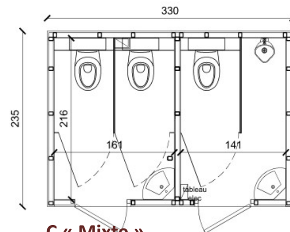
C « Mixte » (3 WC, 1 urinoir, 2 lave main)
