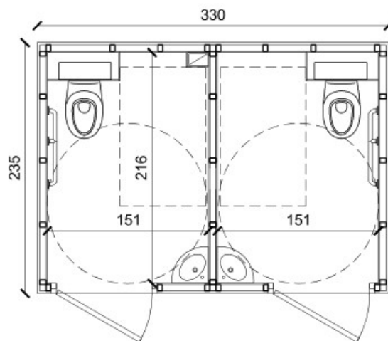
C « PMR » Double (2WC, 2 lave main)
