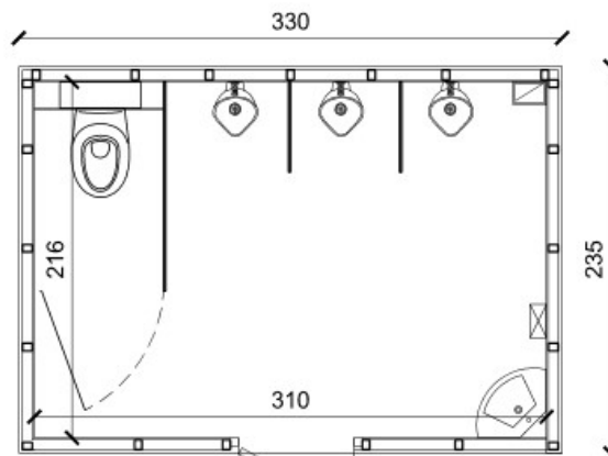
C « Hommes » (1 WC, 3 urinoirs, 1 lave main)
