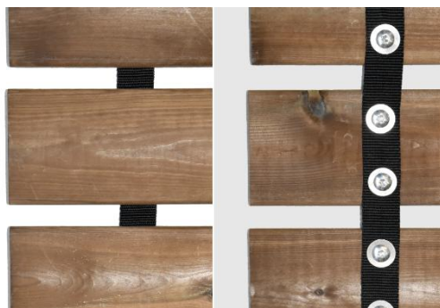
Doghe collegate mediante cinghie in poliestere imputrescibile.
